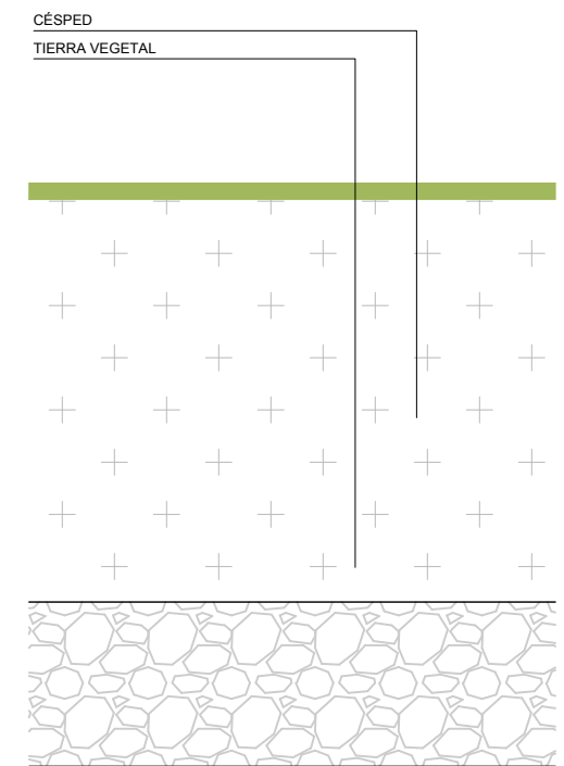
06 SECCIÓN CÉSPED
