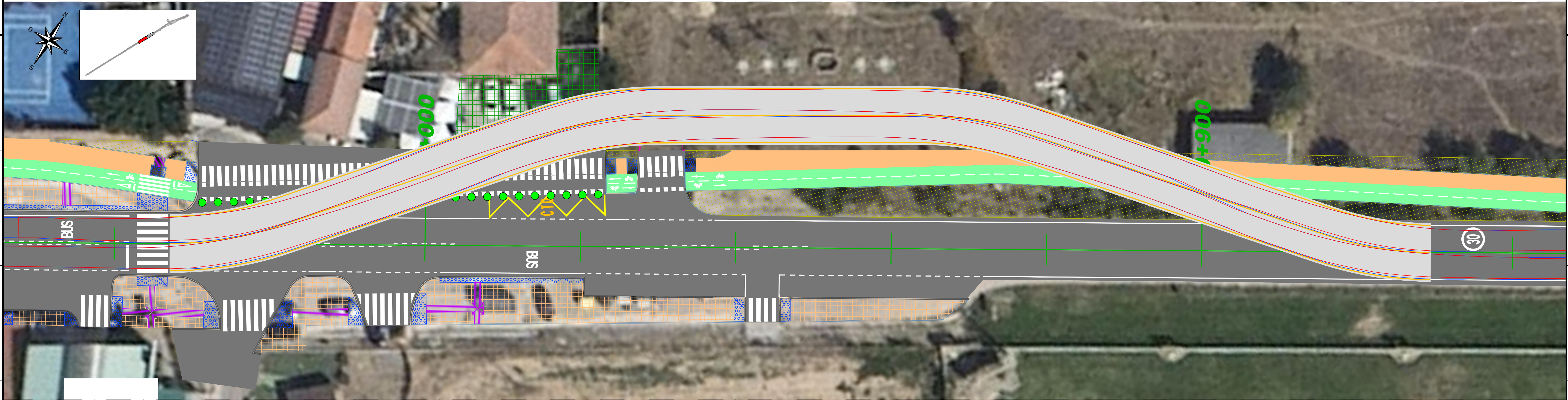
ESTUDIO TRAZADAS E: 1/250 Vehículo patrón: AUTOBÚS RÍGIDO NORMA 3.1 I.C.
