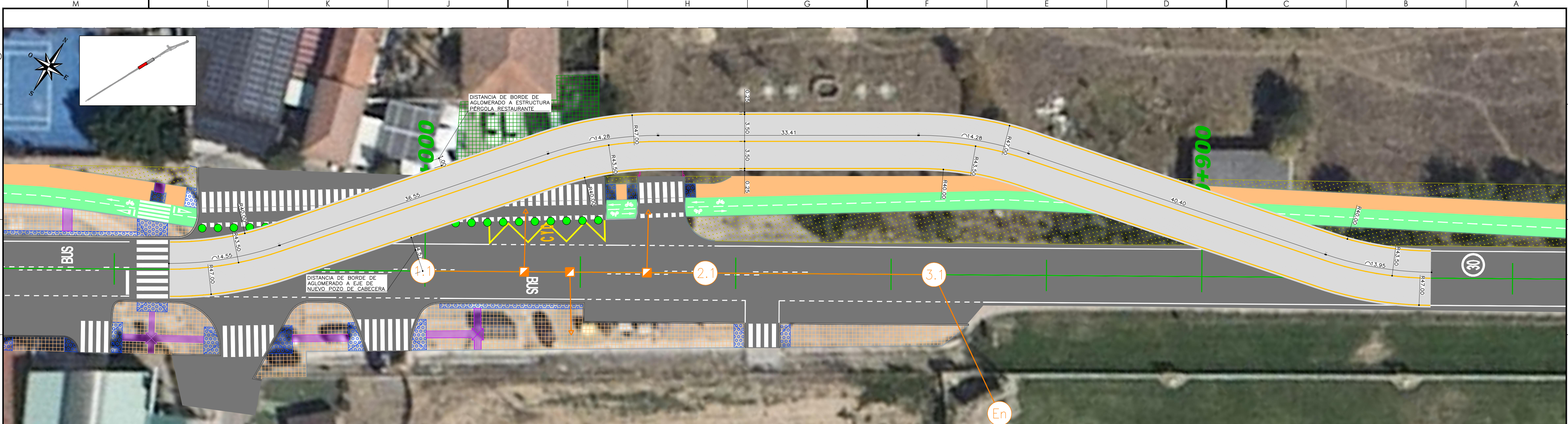
TRAZADO. PLANTA E: 1/250
