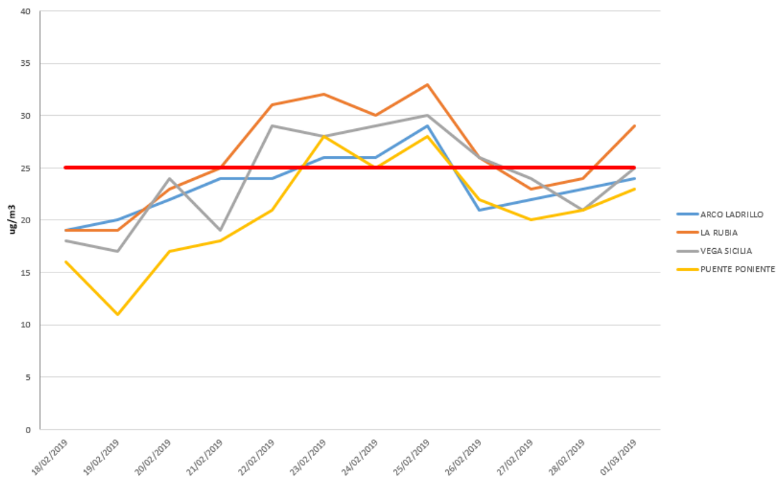
EVOLUCIÓN DIARIA DE PARTICULAS PM2.5
