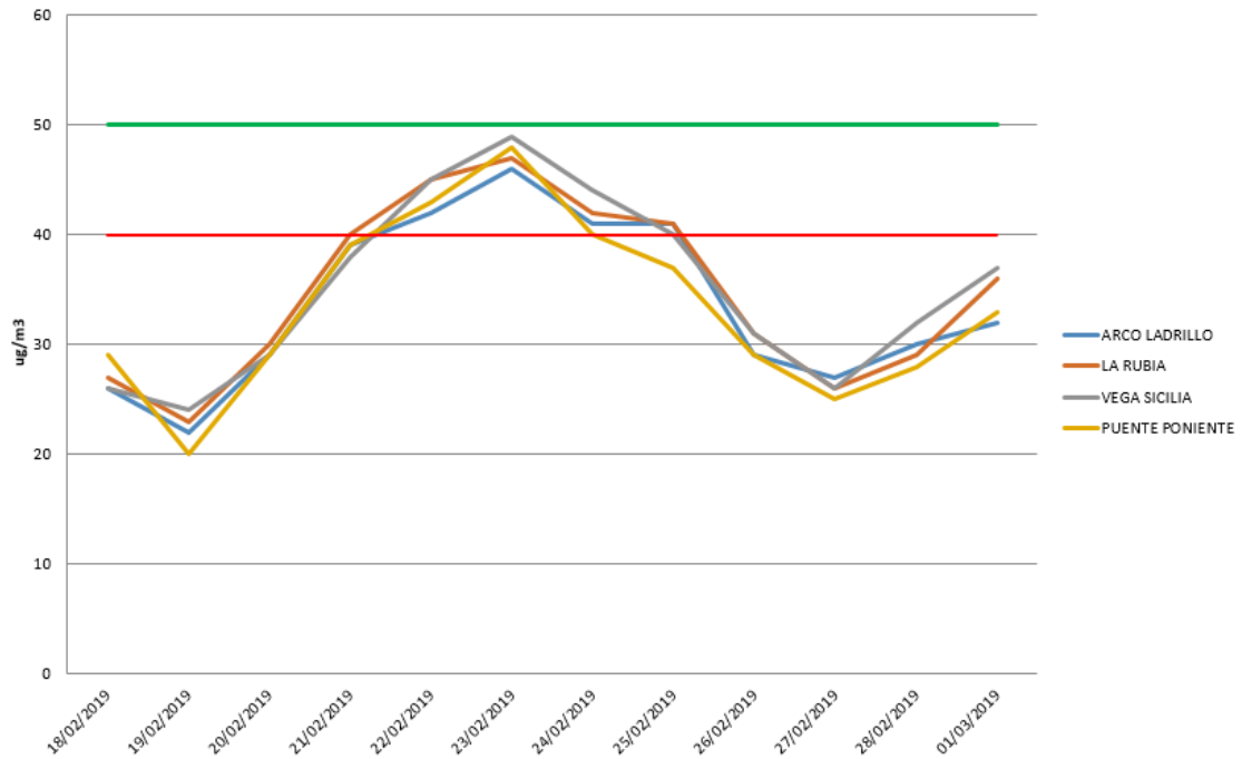
EVOLUCIÓN DIARIA DE PARTICULAS PM10
