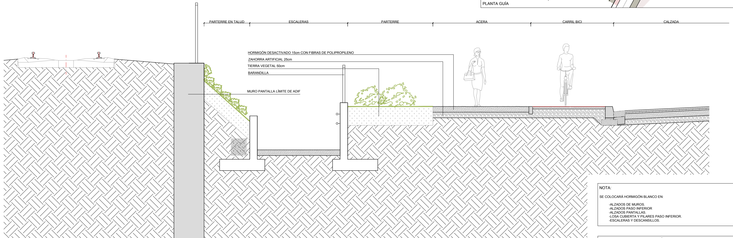
SECCIÓN 7-7 Escala 1/25 Cotas en m
