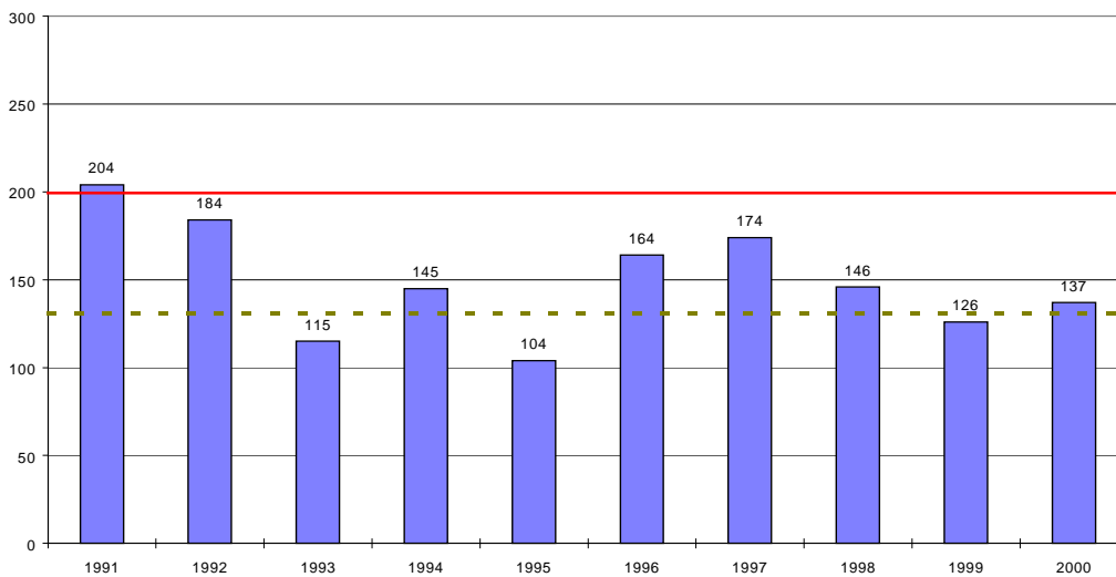
Gráfica 4.3.11 Evolución del percentil 98 para el \text{NO}_2 , frente a los valores límite y guía, Estación Vicente Mortes.
