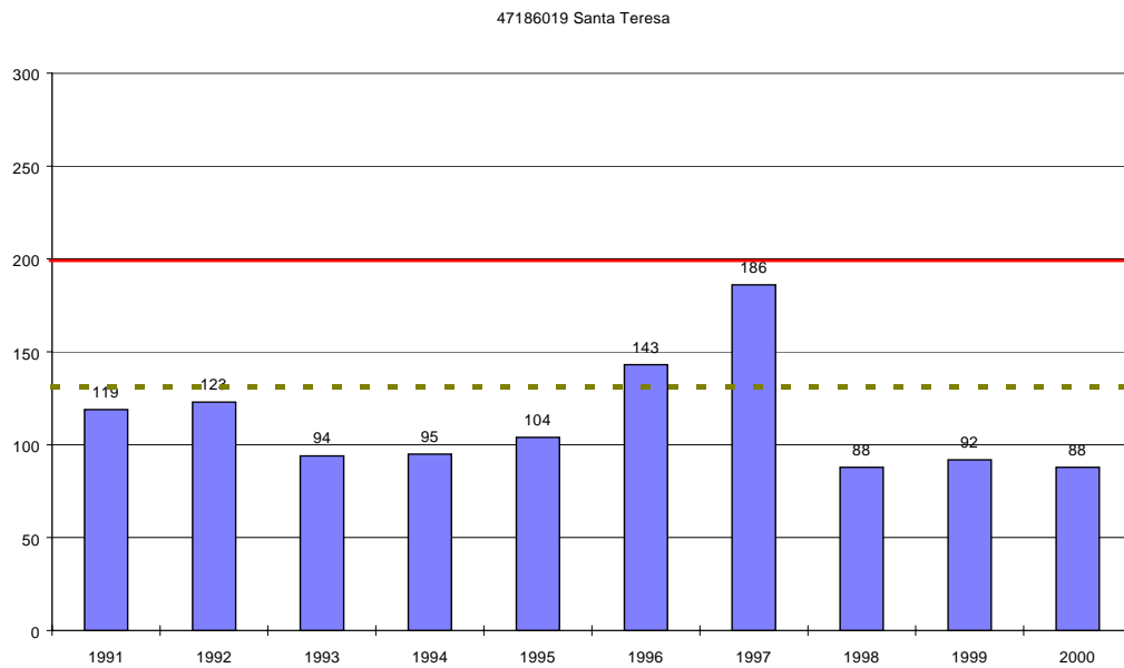
Gráfica 4.3.9 Evolución del percentil 98 para el \text{NO}_2 , frente a los valores límite y guía, Estación Santa Teresa.
