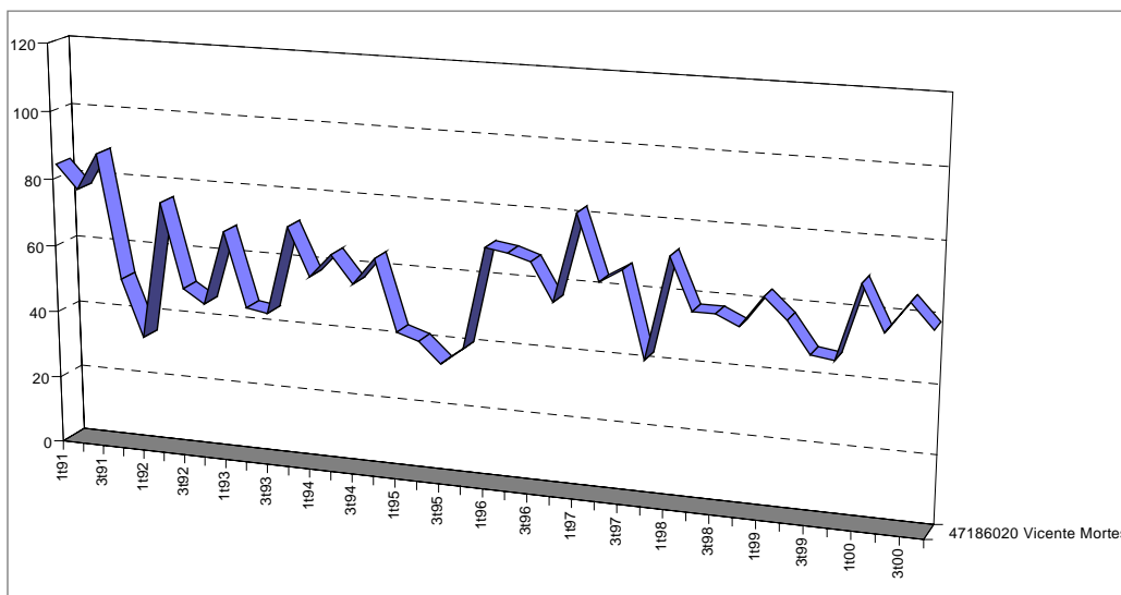
Gráfica 4.3.12 Evolución de las medias trimestrales del \text{NO}_2 Estación Vicente Mortes.
