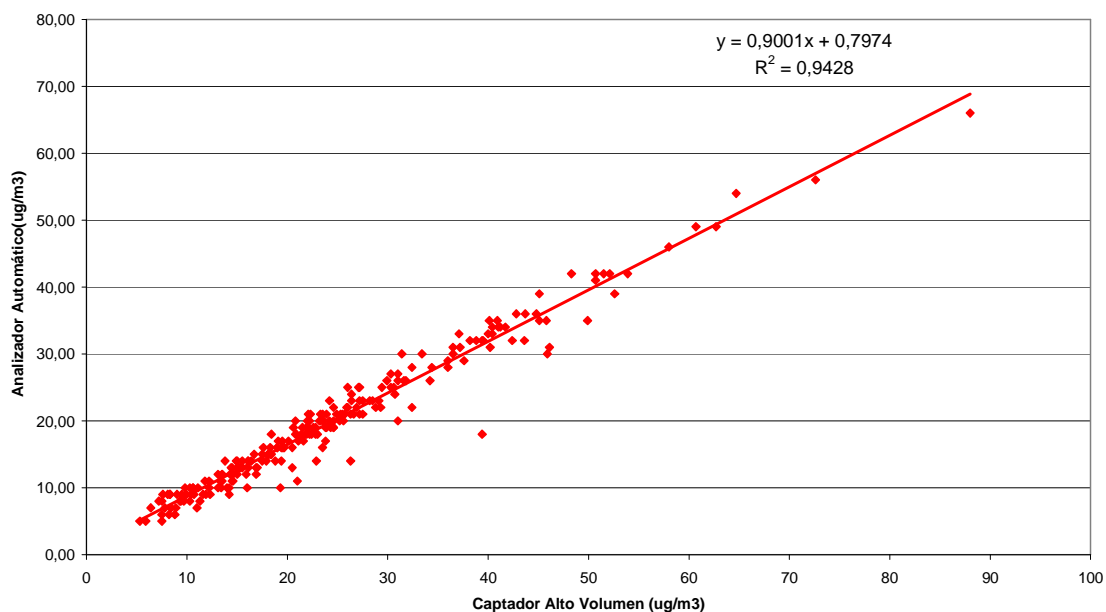
Correlación Partículas PM10 Arco Ladrillo 2
