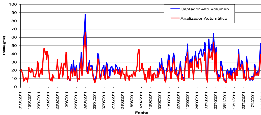
Evolución diaria de partículas PM10 (Arco Ladrillo 2)
