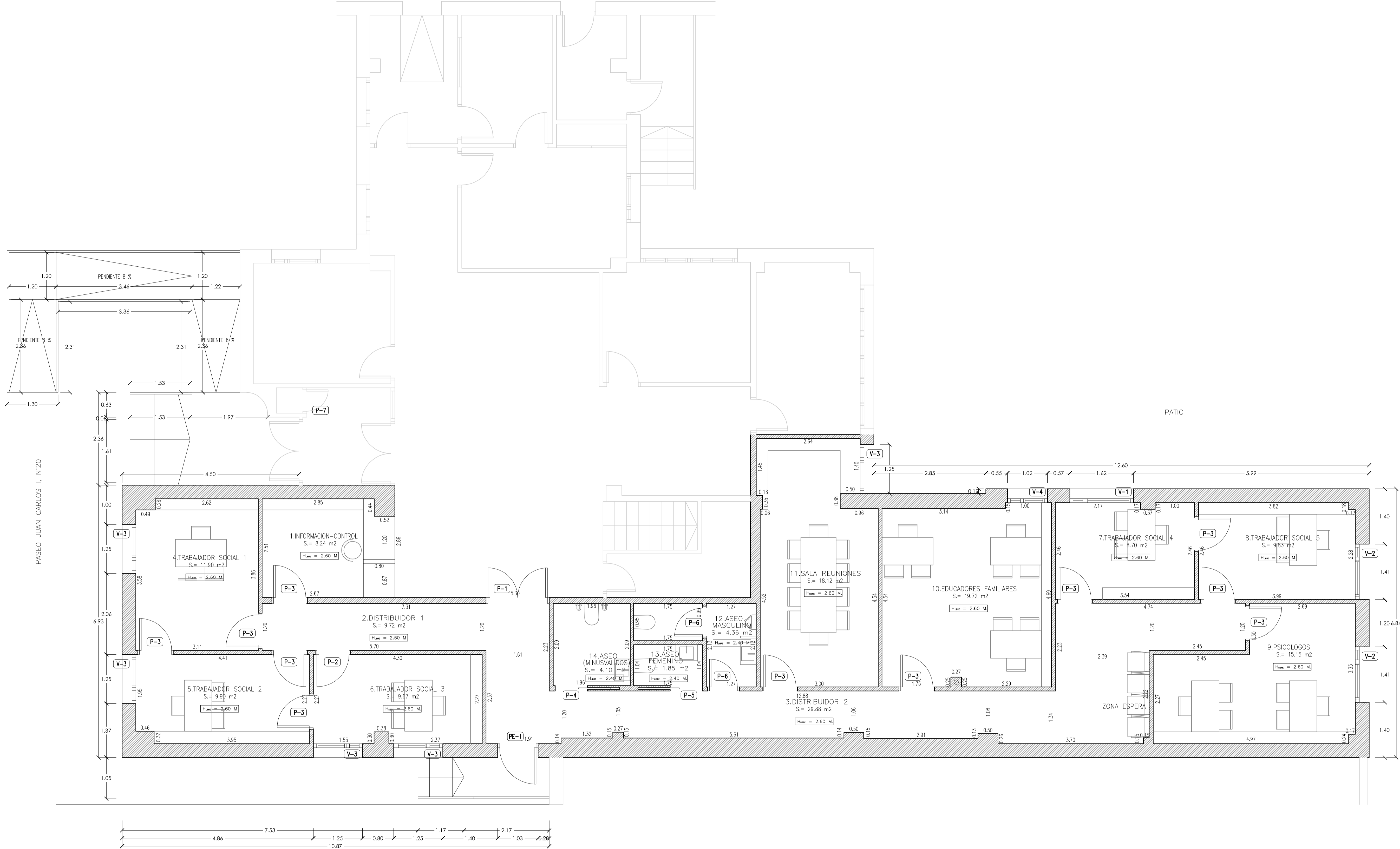
PLANTA BAJA (COTA +0.87)
